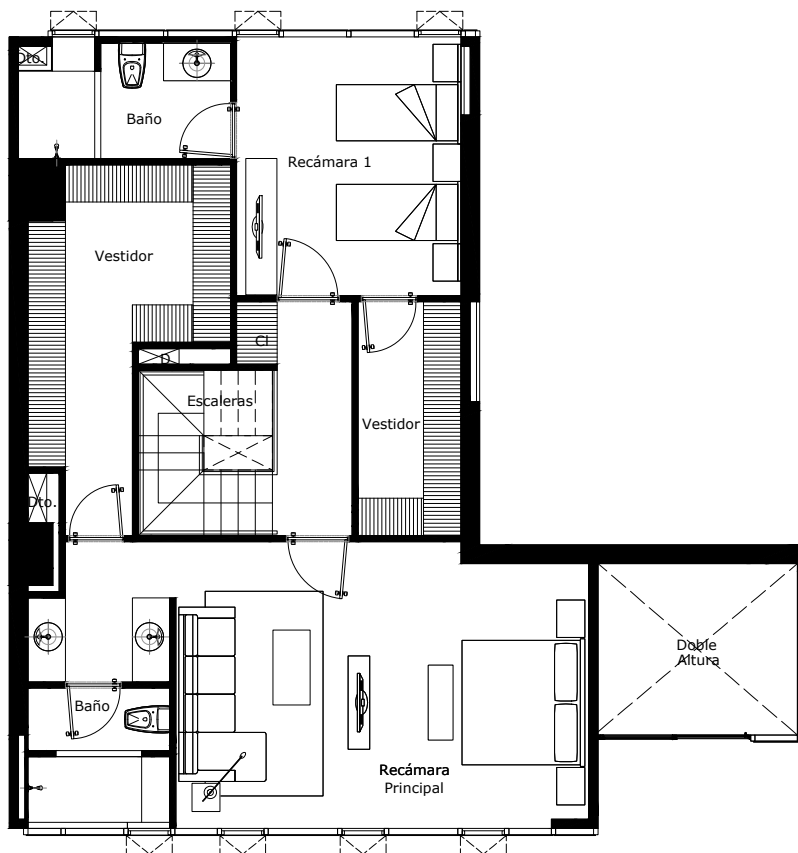
Planta Alta
